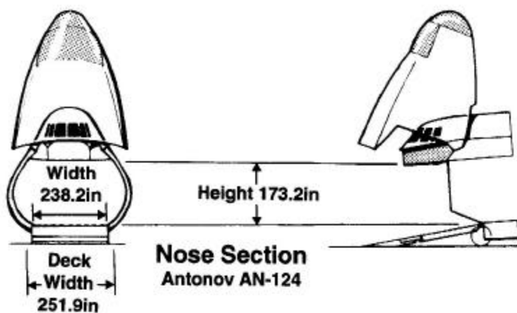
Cargo Door Openings Antonov AN-124
